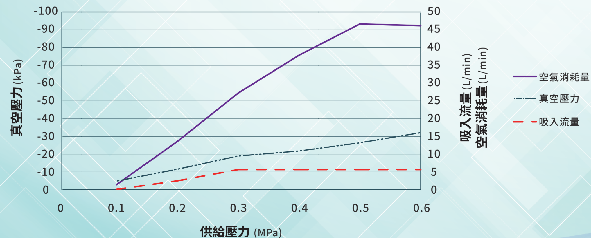
▶ 流量特性
