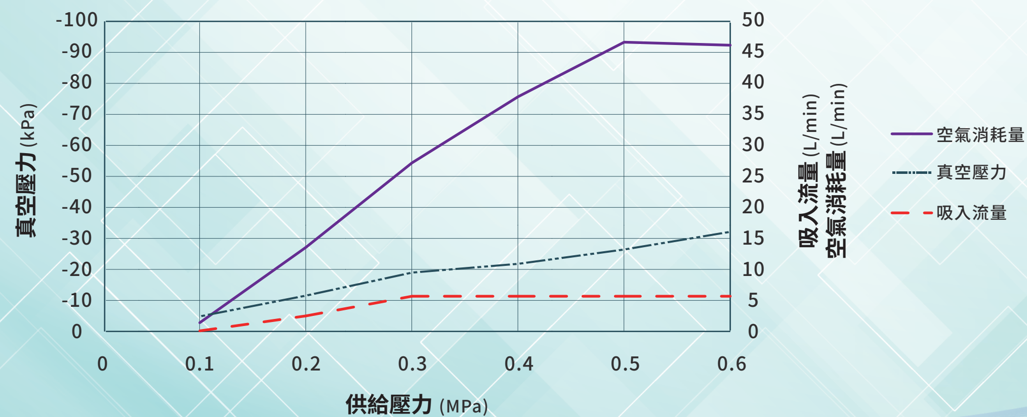
▶ 流量特性
