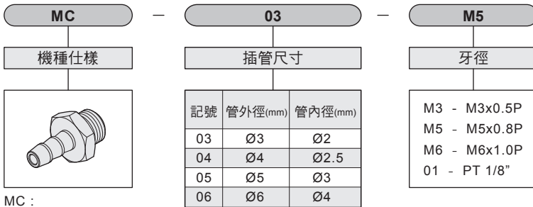
MC : 極小型直立型接頭
