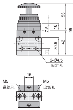
● MV-15- B - 09 連鎖型 / 押入定位 B: 底部配管
