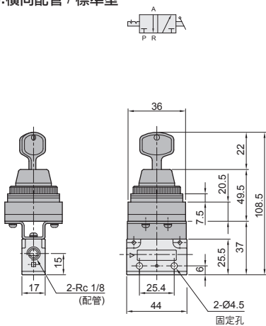
● MV-15- S - 11 鑰匙型 / 旋轉定位 S: 橫向配管 / 標準型
