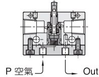
● MV-15B-01 (底部配管/基本型)
