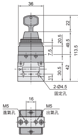
● MV-15- B - 11 鑰匙型 / 旋轉定位 B: 底部配管
