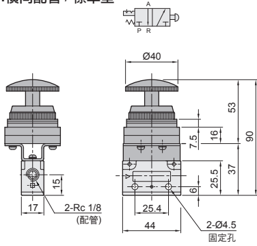
● MV-15- S - 09 連鎖型 / 押入定位 S: 橫向配管 / 標準型
