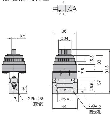
● MV-15- S - 10 選擇型 / 旋轉定位 S: 橫向配管 / 標準型
